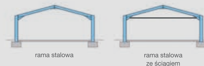
Konstrukcja ramowa stalowa ocynkowana bez ściągu, dach pokryty dachówką, okładzina ścienna z drewna.
